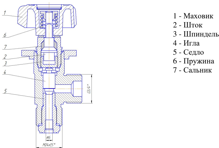
Рис.2 Устройство клапана К-2103-400, К-2103-16
